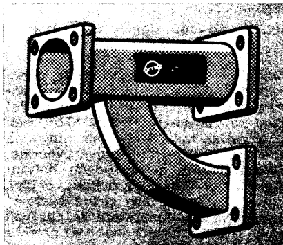
Obr. 11. Vlnovodná výhybka — vlevo vstup, vpravo nahore výstup vodorovně a dole výstup svisle polarizovaného signálu
